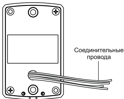
Рисунок 10 - Назначение проводов считывателя
